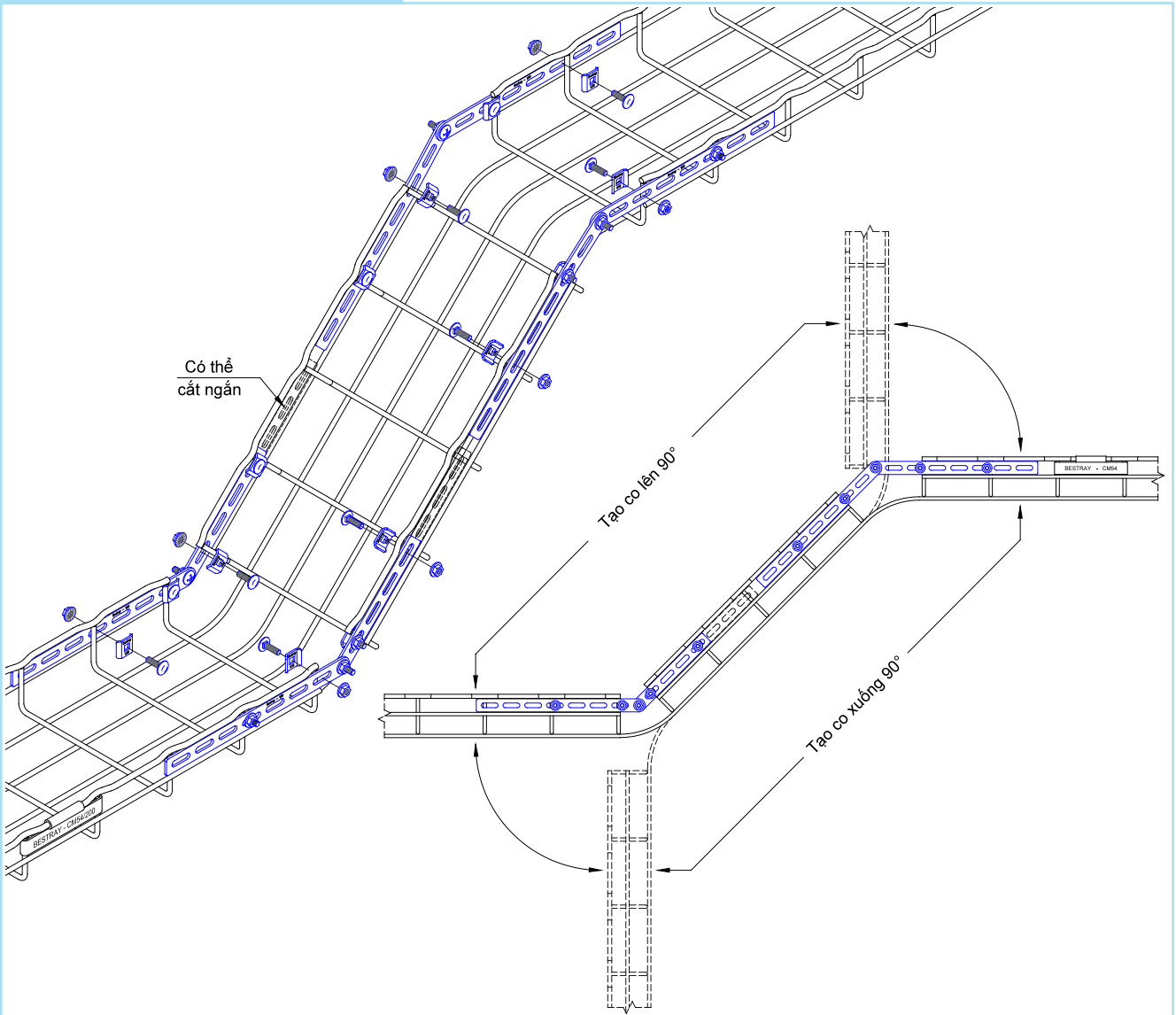
Tạo Co Lên và Xuống (Co Chữ Z)
