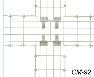
Ngã Tư (Góc Vuông)
