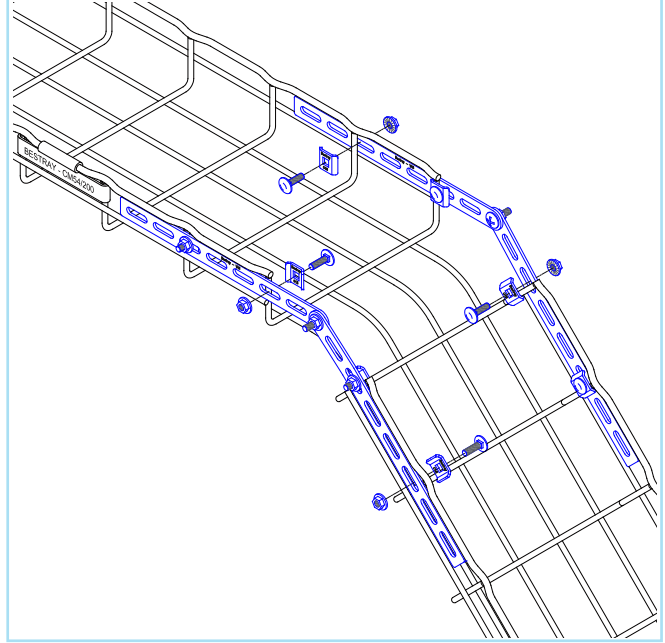
Tạo Co Xuống (0~90°)
