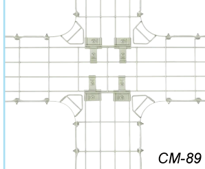
Ngã Tư (R=75mm)
