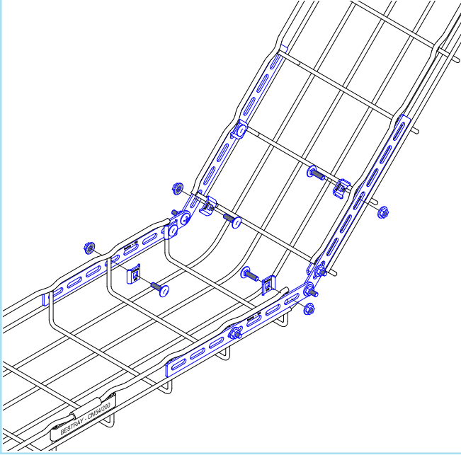
Tạo Co Lên và Xuống (Co Chữ Z)
